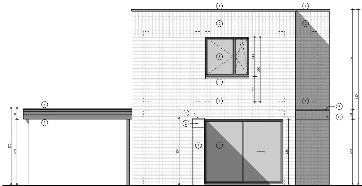
NT VOORGEVEL
