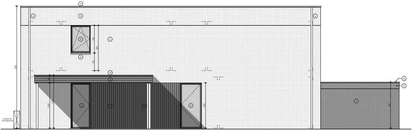
NT LINKER ZIJGEVEL
