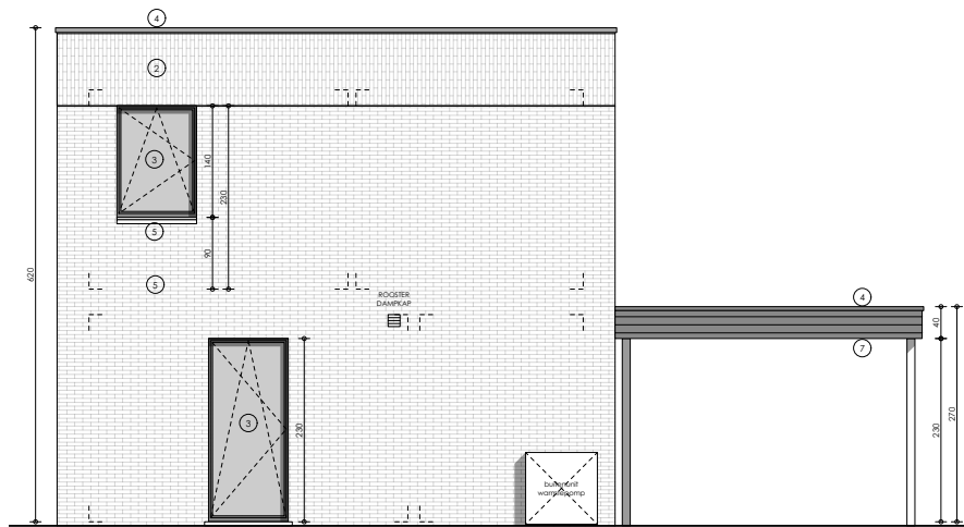
NT ACHTERGEVEL
