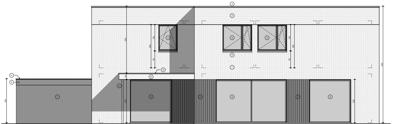
NT RECHTER ZIJGEVEL
